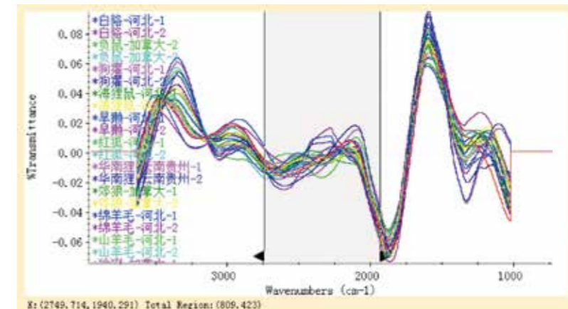
红外光谱鉴别毛纤维的化学计量过程
