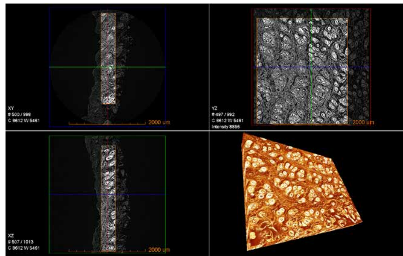
皮革的Micro CT 三维扫描切面测量
