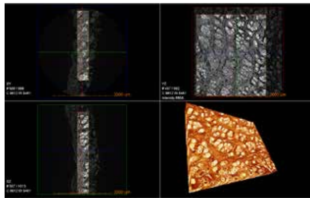
皮革的Micro CT 三维扫描切面测量
