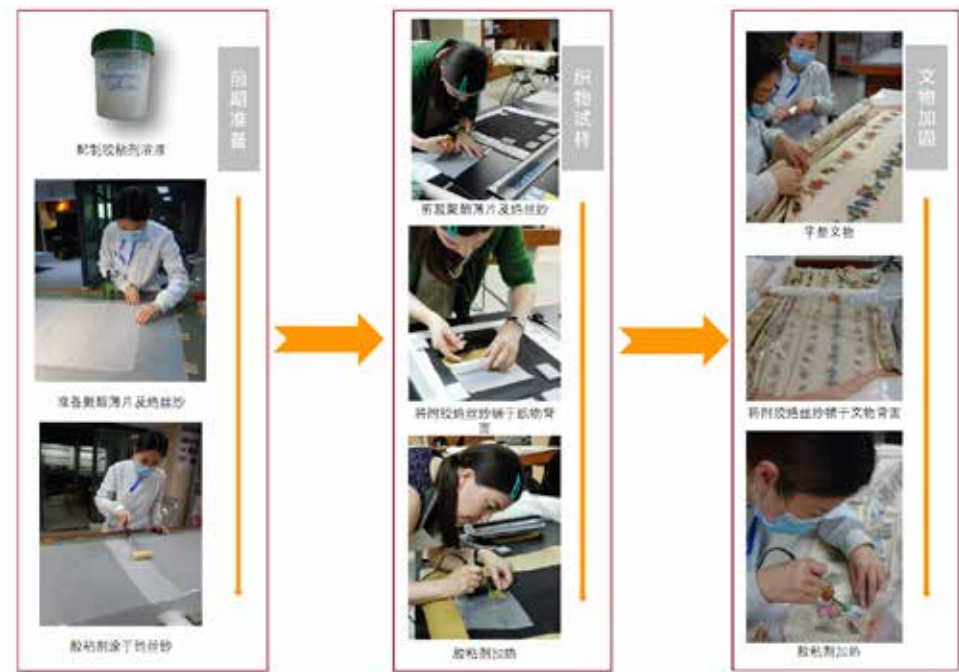
胶粘剂加固工艺流程
